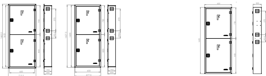
جعبه آتش نشانی دوکابین عمودی
